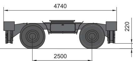
Sottocarro con 4 stabilizzatori
